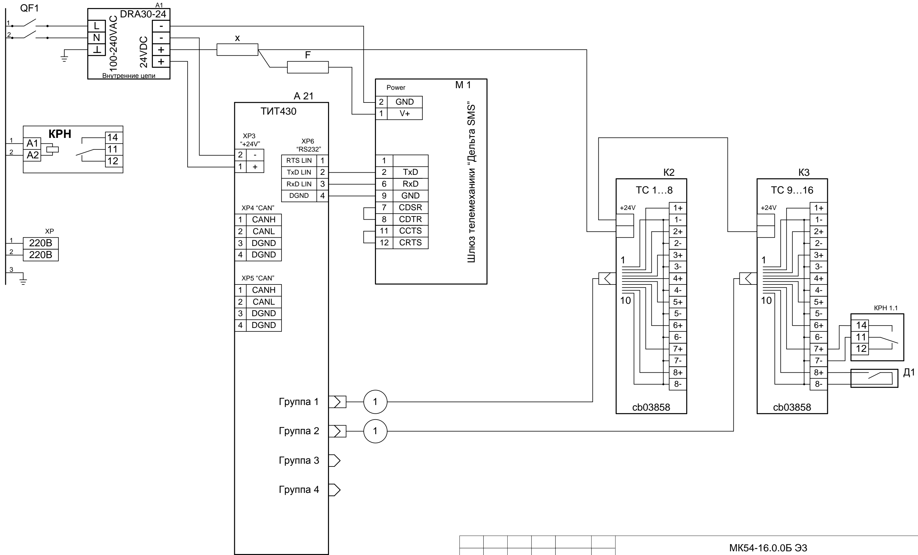
Схема кабеля 1
